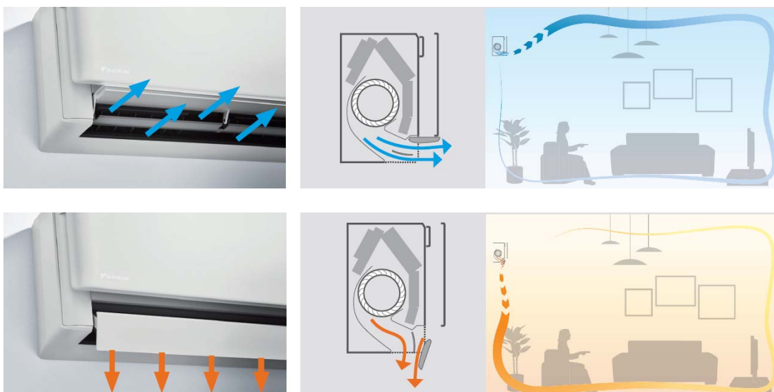
Na vrhu je prikazan primjer Coanda efekta u načinu rada za hlađenje (stropni protok zraka), a donja slika prikazuje Coanda efekt u načinu rada za zagrijavanje (vertikalni protok zraka).
